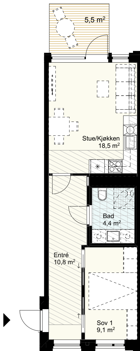
Generell himlingshøyde 2,6m Nedføret himling fra min. 2,2m
