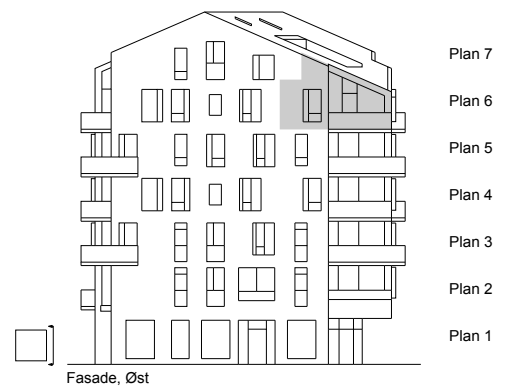
Fasade, Øst
